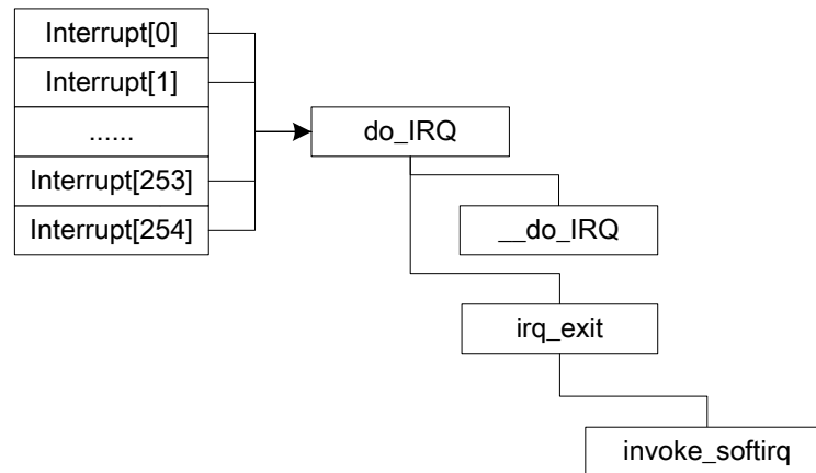
图表 2-8 do_IRQ 函数调用树
