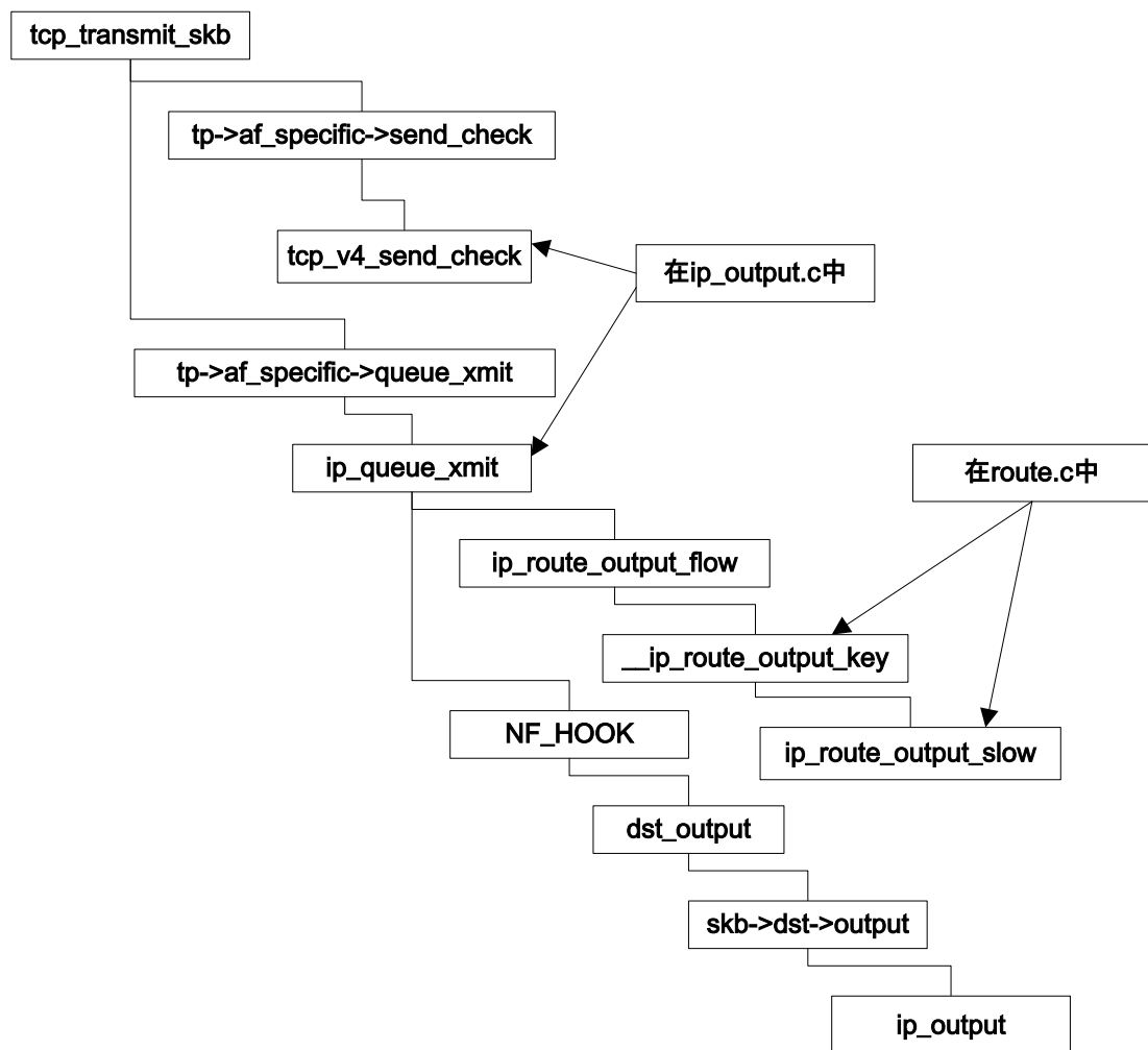
图表 5-16tcp_transmit_skb 调用树
