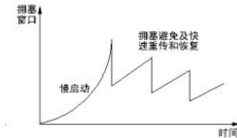
图表 5-20(b) 快速重传和快速恢复
