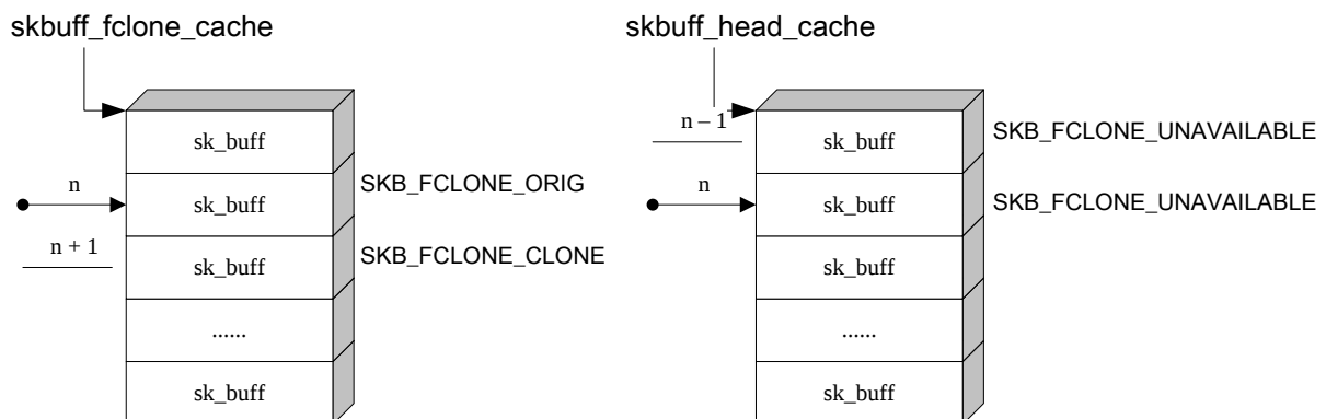
图表 2-14 不同 skb cache 中的内存操作
