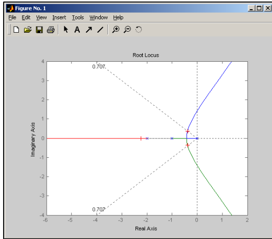
图 6.20 (a) 等 ζ 线和等 ω n 线
