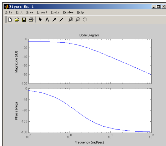
图 6.14 (a) Bode 图
