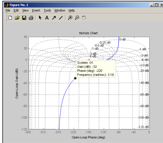
图 6.16 nichols 图
