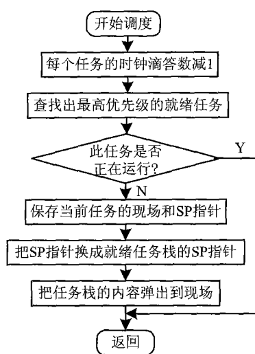
图3 任务调度流程
