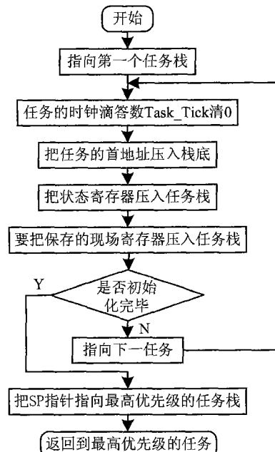
图2 任务初始化流程
