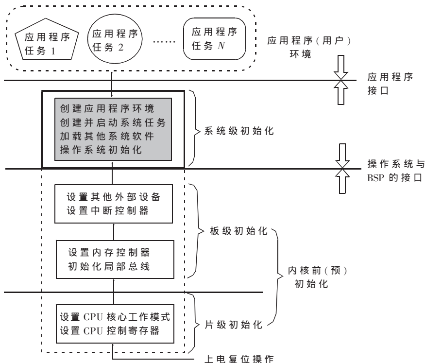
图 3 嵌入式系统的初始化过程及 BSP 的功能
