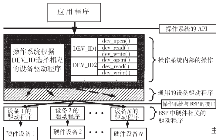
图4 系统调用、通用设备驱动程序与BSP之间的关系
