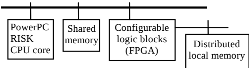
Fig.3 Abstract model of target architecture 图3 目标系统结构抽象模型
