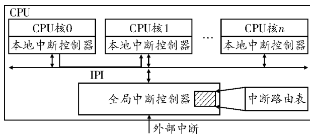
图 4 多核中断系统
