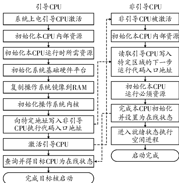
图1 多核操作系统非引导 CPU 启动过程
