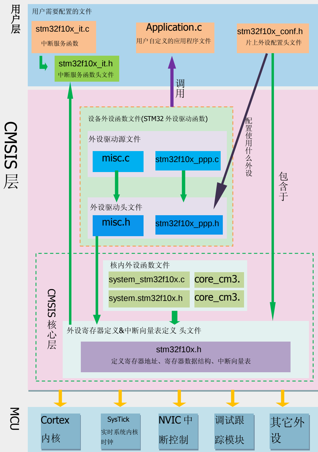
图 0-6 描述了 STM32 库各文件之间的调用关系，这个图省略了 DSP 核 (Cortex-M3 没有 DSP 核) 和实时系统层部分的文件关系。在实际的使用库开发工程的过程中，我们把位于 CMSIS 层的文件包含进工程，丝毫不需修改，也不建议修改。
